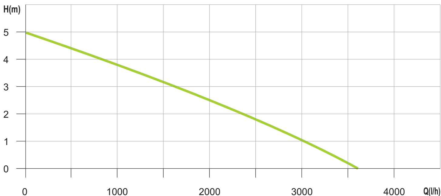
Dijagram protoka
